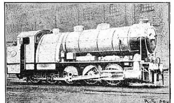
Fig. 1.—Nuevo tipo de locomotora de la Great Eastern Railway Co.
